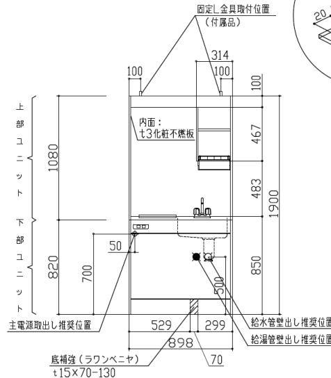
A正面図
