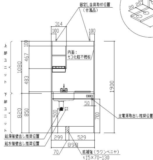
A正面図
