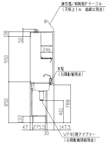
D側面図
