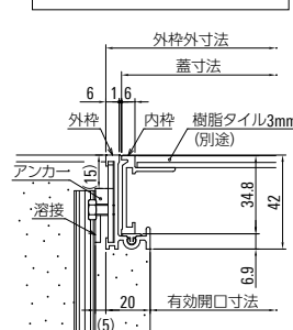
樹脂タイル仕様 (Pタイル)
