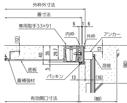
モルタル充填仕様
