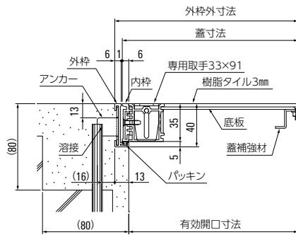
樹脂タイル仕様 (Pタイル)
