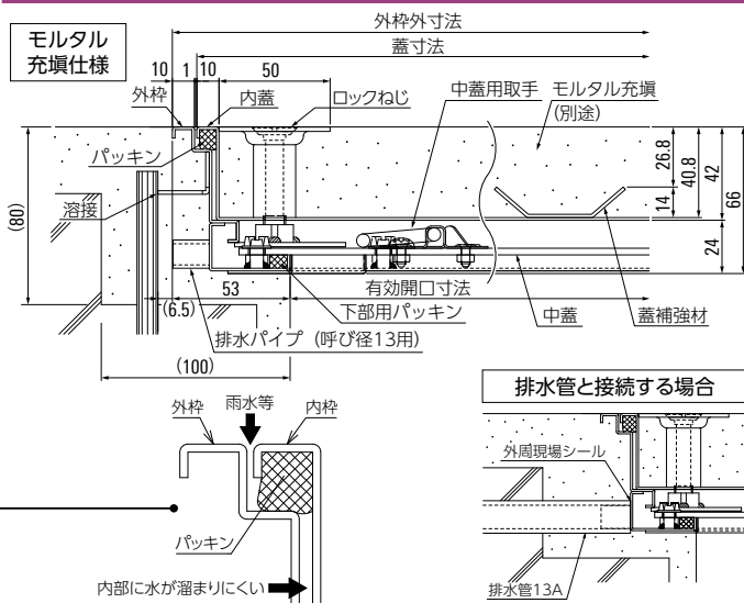
納まり図
