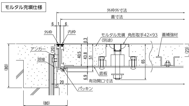
納まり図
