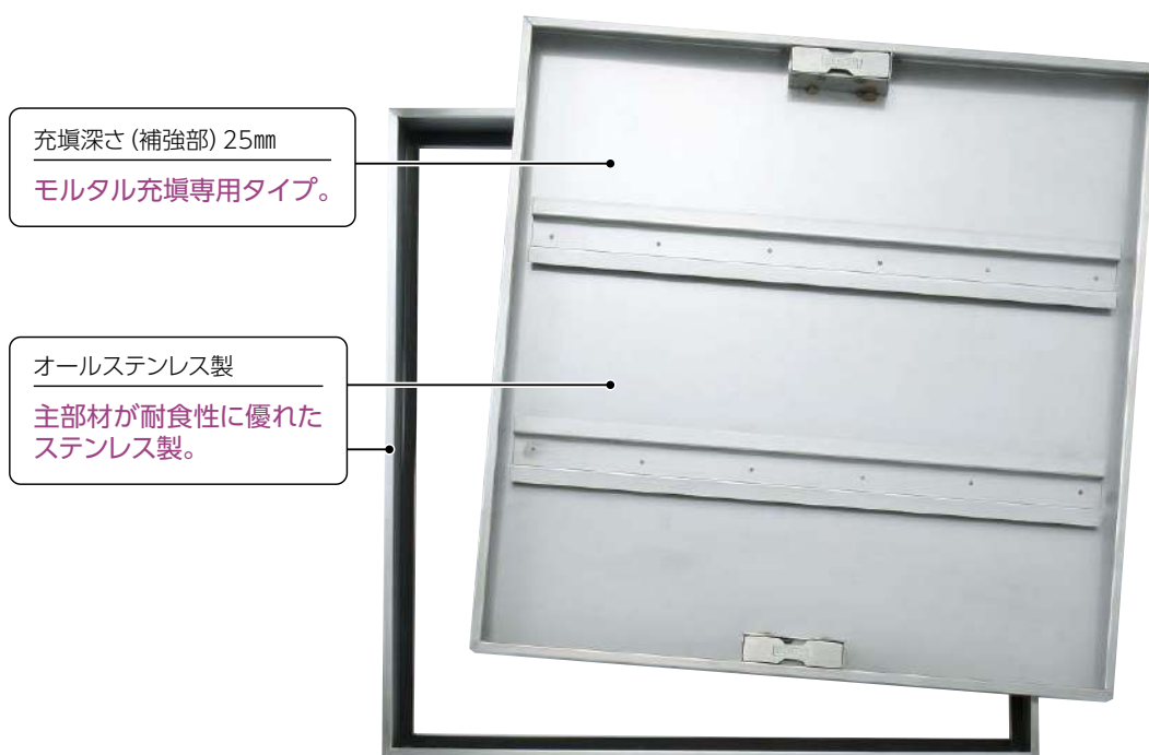
部材仕様
