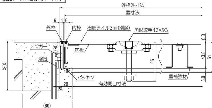
樹脂タイル仕様 (Pタイル)
