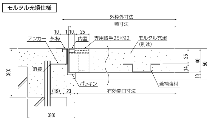
納まり図
