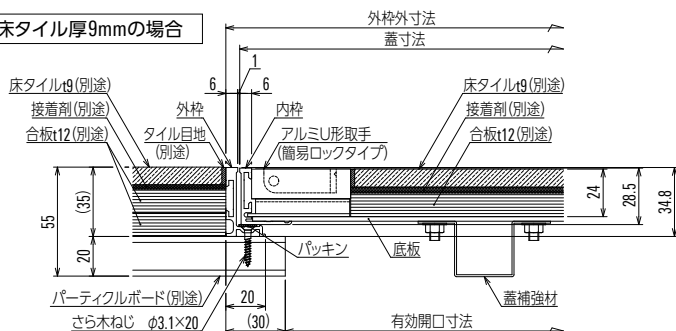
木製下地納まり図
