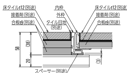
部材仕様
