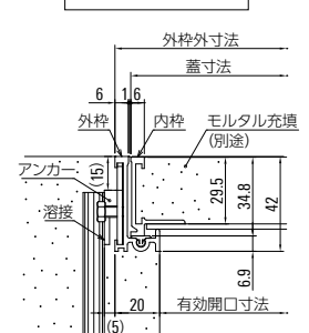
モルタル充填仕様
