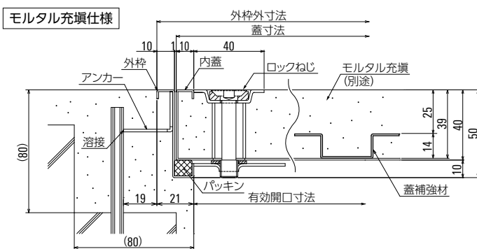
納まり図
