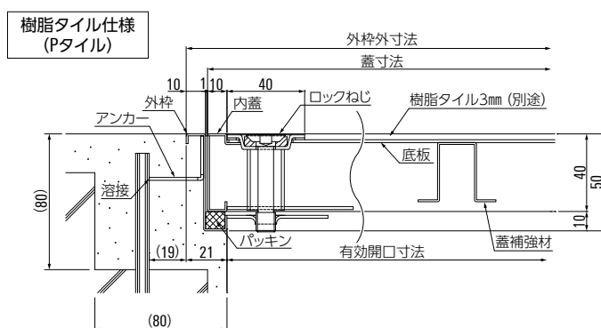
納まり図
