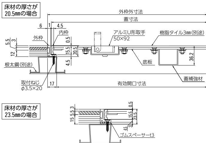
納まり図
