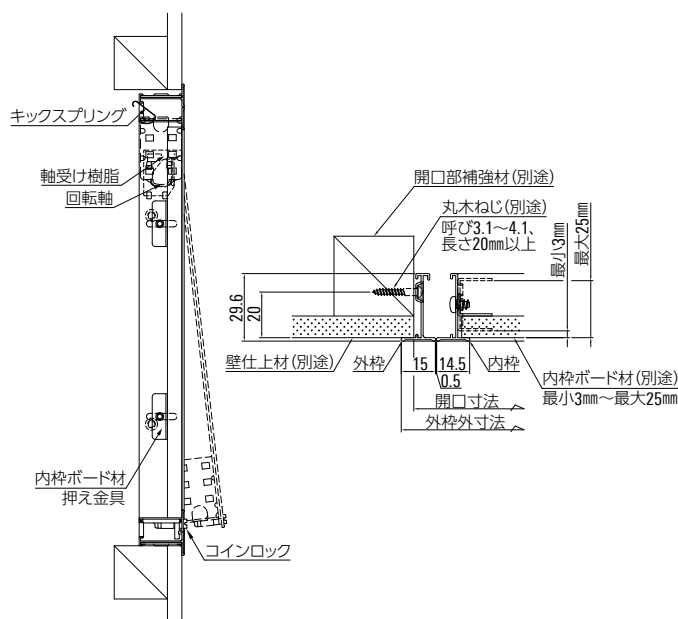
納まり図
