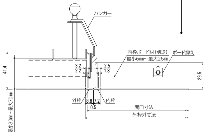
納まり図
