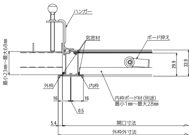
納まり図
