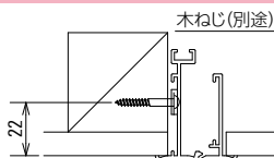
木下地納まり図
