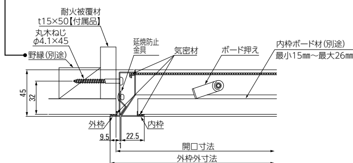
納まり図
