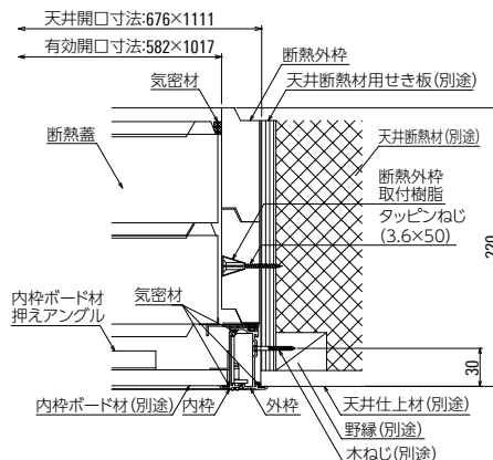
■詳細図
