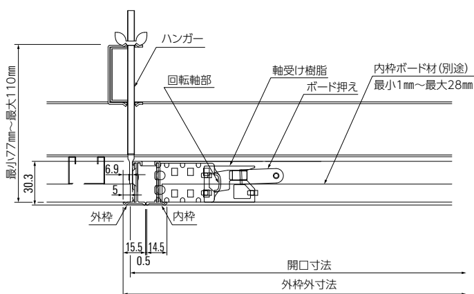
納まり図
