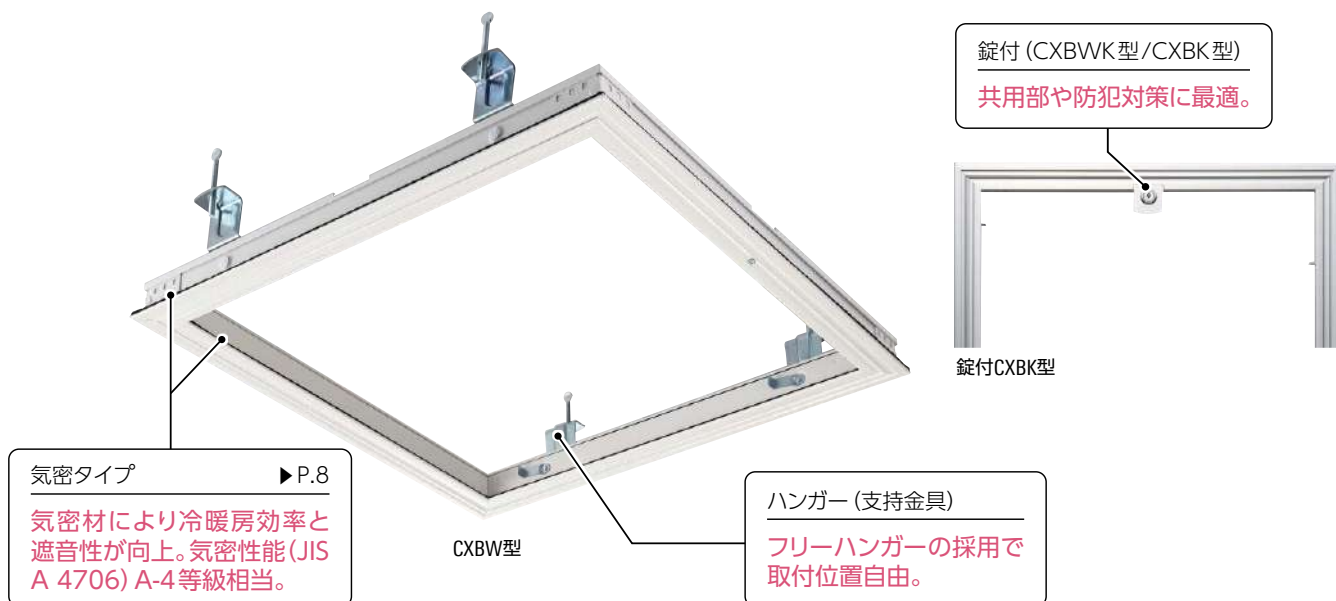
納まり図
