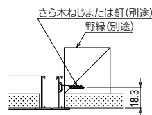
木下地納まり図
