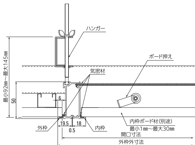
納まり図
