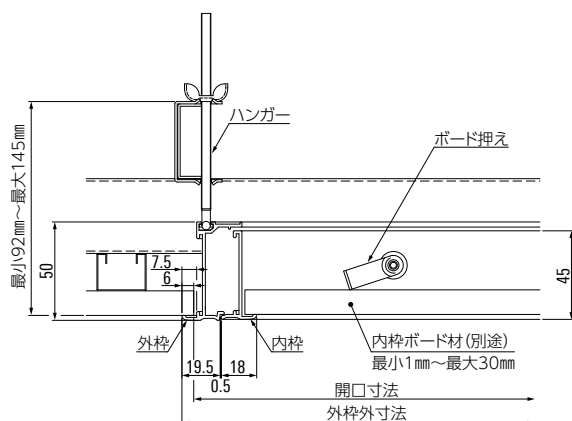
納まり図
