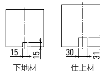
●錠付(特注品)
