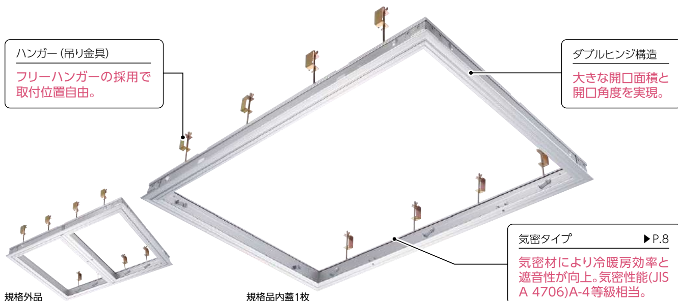
納まり図
