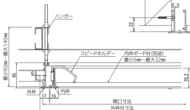
納まり図
