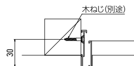
木下地納まり図
